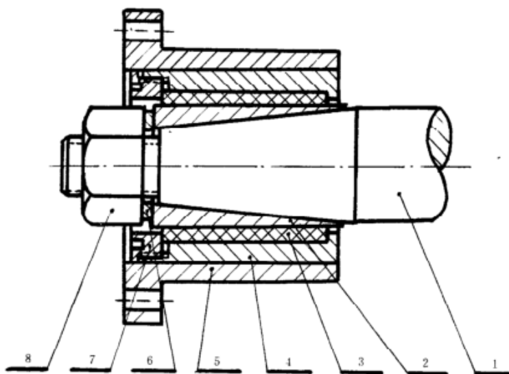
图4 钢轴套和塑料轴承安装图
