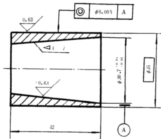
图 3 钢轴套
