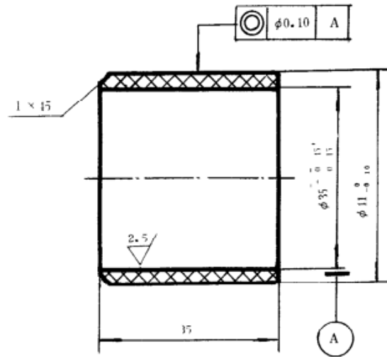
图 2 塑料轴承
